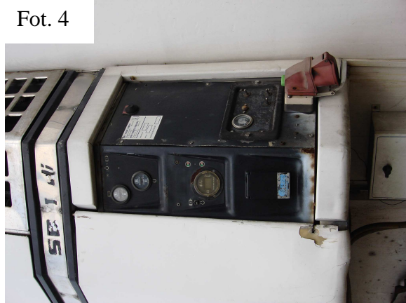
Fot. 3,4 Widok agregatu (urządzenia chłodniczego) THERMO KING SB II Di
